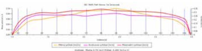
■ Rozložení rychlostí v profilu.
